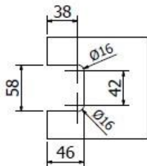
Výrez do skla s tesnením 8861
