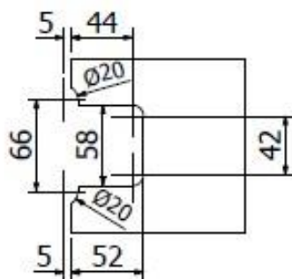
Výrez do skla bez tesnenia
